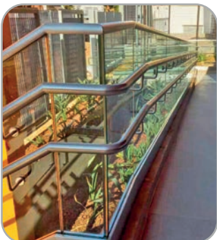
Guarda-Corpo em Vidro Acabamento Perfil "U"
